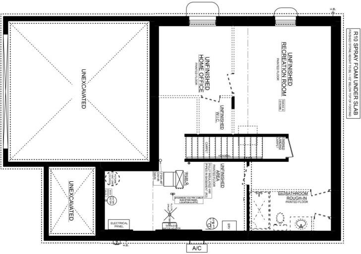
OAKMONT 'C' BASEMENT PLAN
