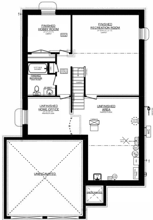
GLENWOOD 'B' BASEMENT PLAN
